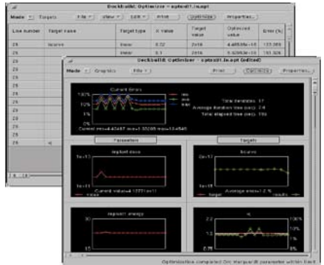
DeckBuild로 제어되는 옵티마이저는 공정 변수를 최적화하여, 사용자가 정의한 타겟(예를 들어, v_t 또는 SIMS 프로파일)에 도달할 수 있습니다.
